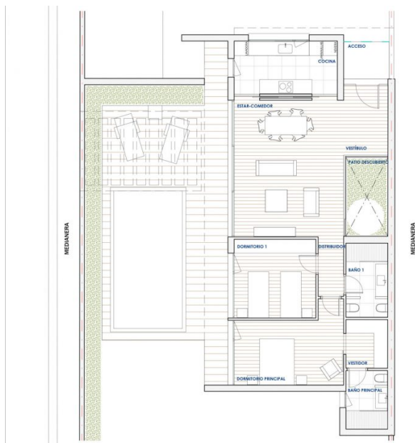
PLANTA BAJA - VIVIENDA TIPO I
